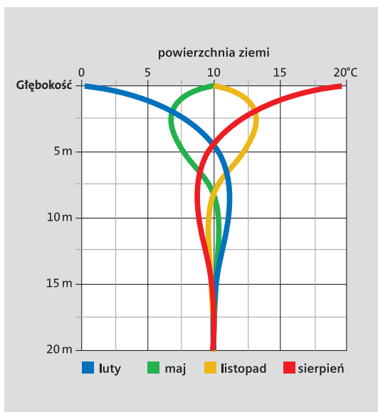
Przebieg temperatury rocznej gruntu jako źródła ciepła
